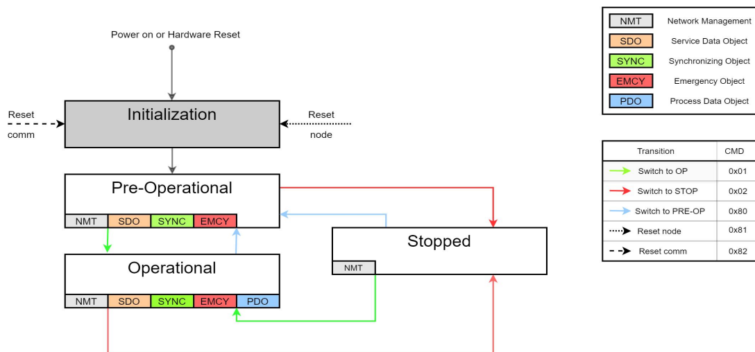
图 3-1 NMT 状态机
